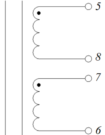
Электрическая схема
