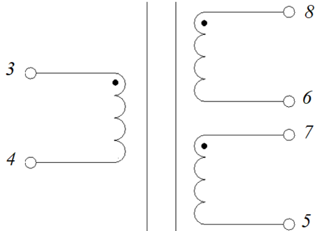
Электрическая схема
