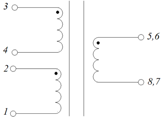
Электрическая схема
