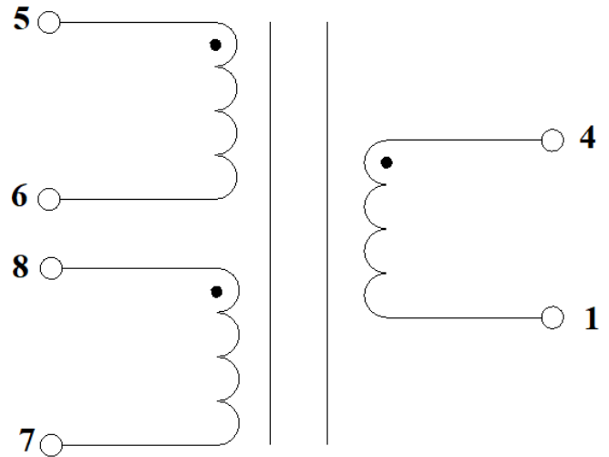
Электрическая схема
