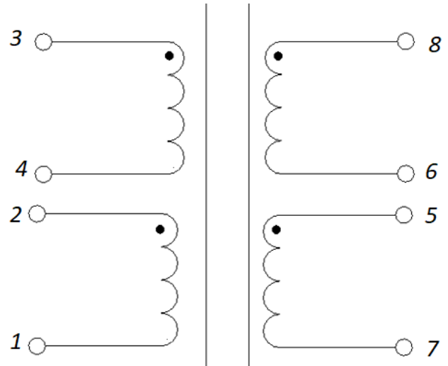
Электрическая схема
