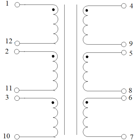
Электрическая схема
