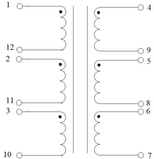
Электрическая схема
