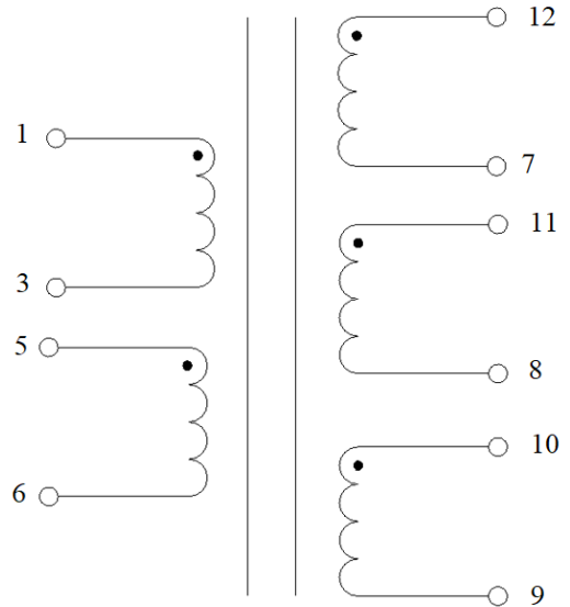
Электрическая схема
