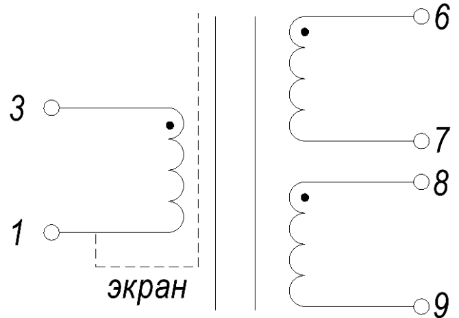
Электрическая схема
