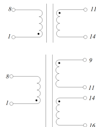
Электрическая схема
