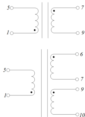
Электрическая схема
