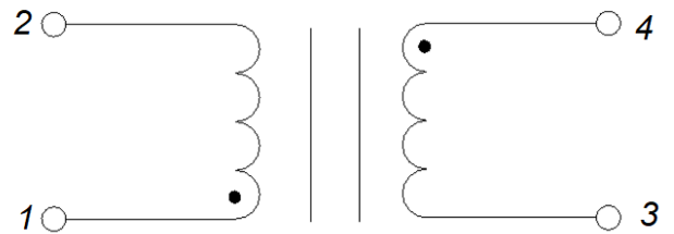
Электрическая схема
