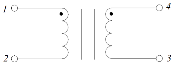
Электрическая схема
